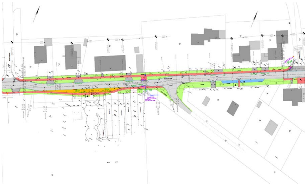
Planung 2. Bauabschnitt Quelle: Keese ingenieure + planer
