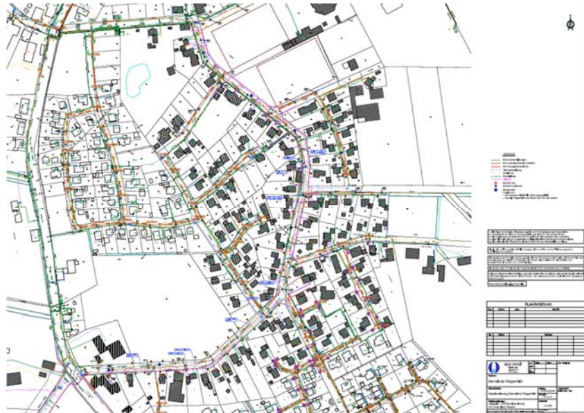
Lageplan „Am Entenplatz“ Quelle: aqua consult
